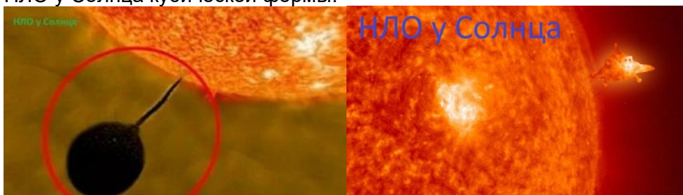
НЛО огромных размеров (диаметр НЛО ~ 200 тыс км.) у Солнца.
