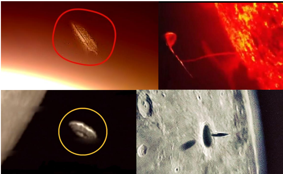
НЛО огромных размеров у Солнца. НЛО на Луне Значит в космосе есть высокоразвитые цивилизации.
