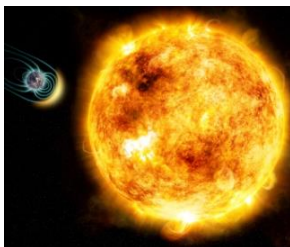
Солнце и Земля
